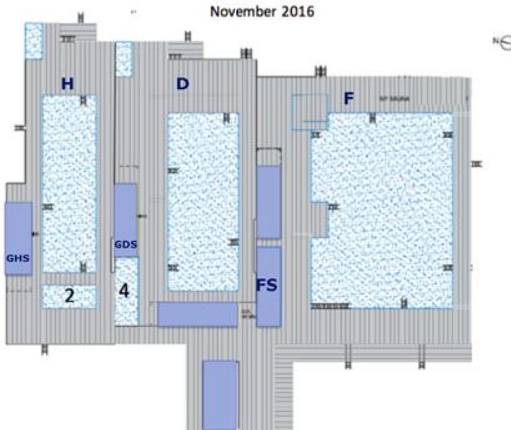
Figur 1: Der stilles forslag om, at herre-, dame- og fællesafdelingen, som de fremstod i 2016 fortsat skal eksistere som ovenstående tegning viser. Saunaen i byggefelt 2 skal være en suveræn herresauna, og saunaen i byggefelt 4 skal være en suveræn damesauna. Fra 1. Maj til 30 September Bruges Saunaen i byggefelt 2 til fællessegmentet Fra kl. 08:00 – 10:00 & 19:00 – 22:00.
